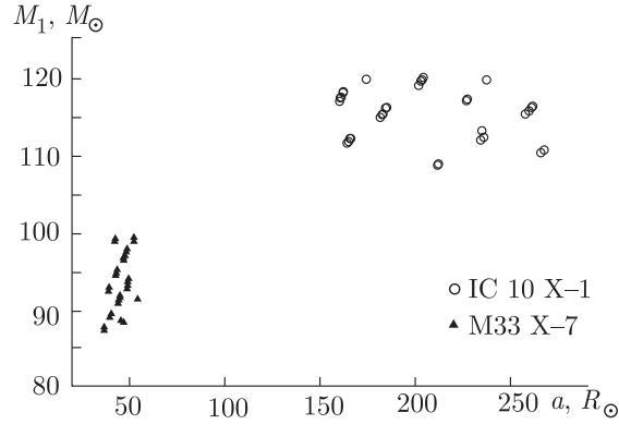
Рис. 206. Начальные параметры систем, результатом эволюции которых являются исследуемые двойные системы: по оси ординат — начальная масса первичной (изначально более массивной) компоненты, по оси абсцисс — начальная большая полуось системы. Треугольниками обозначены двойные системы, эволюция которых приводит к образованию систем типа M 33 X-7, кружками — двойные системы, эволюция которых приводит к образованию систем типа IC 10 X-1. Значения свободных параметров задачи приняты следующими: \alpha = 0,1 , k_{WR} = 0,1 , k_{bh} = 0,3
