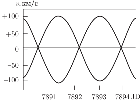
Рис. 7. Кривые лучевых скоростей обеих компонент спектрально-двойной системы BV241
