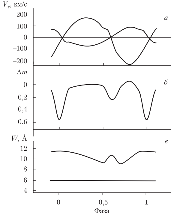
Рис. 55. Теоретические кривые лучевых скоростей (а), кривая блеска (б) и эквивалентные ширины линии H_\gamma двух звезд (в) для тестовой модели. На нижнем рисунке кривая соответствует звезде с температурой T_1 = 10\,000\text{ К} , прямая — T_2 = 15\,000\text{ К} . Параметры модели: M_1 = 4M_\odot , M_2 = 10M_\odot , P = 5^d , e = 0,15 , \omega = 180^\circ , i = 80^\circ , \mu_1 = \mu_2 = 1 , T_1 = 10000\text{ К} , T_2 = 15000\text{ К} , \psi_0 (фаза периастра) = 0,798
