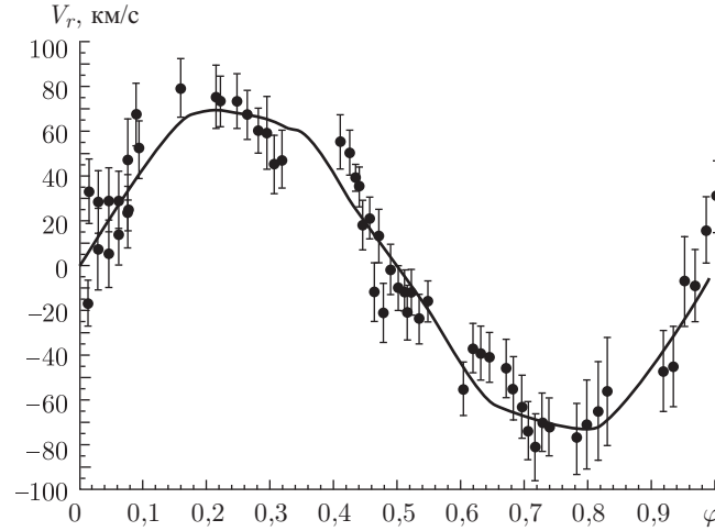
Рис. 187. Наблюдаемая и теоретическая кривые лучевых скоростей оптической звезды в рентгеновской двойной системе HZ Her X-1. Точки — значения лучевой скорости HZ Her из работы (Reynolds et al., 1997). Сплошная линия — теоретическая кривая лучевых скоростей в модели Роша, вычисленная точным алгоритмом при массе компактного объекта m_x = 0,81 M_\odot , массе оптической звезды m_v = 1,80 M_\odot и наклоне орбиты i = 88^\circ
