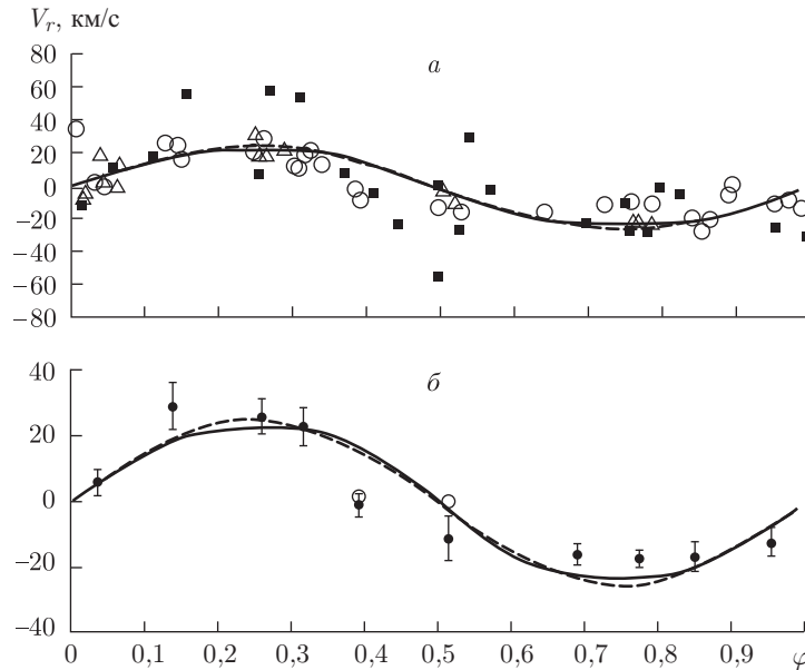
Рис. 169. a — сводная наблюдаемая кривая лучевых скоростей рентгеновской двойной системы SMCX-1. Здесь темными квадратами представлены спектральные данные 1973 г. из работы (Osmer and Hiltner, 1977), светлыми кружками — спектральные данные 1976 г. из работы (Hutchings et al., 1977), светлыми треугольниками — спектральные данные 1989 г. из работы (Reynolds et al., 1993). Для сравнения приведены теоретические кривые лучевых скоростей в модели Роша (сплошная линия) и модели точечных масс (штриховая линия) для массы m_x = 1,48M_\odot , соответствующей минимуму невязки в модели Роша. б — лучевые скорости, усредненные внутри фазовых интервалов (темными кружками представлена средняя интенсивность в фазовом интервале, светлыми — лучевые скорости, исправленные за нормированную функцию анизотропии звездного ветра оптической звезды). Для сравнения, приведена теоретическая кривая лучевых скоростей в модели Роша (сплошная линия) и в модели точечных масс (штриховая линия) для m_x = 1,48M_\odot
