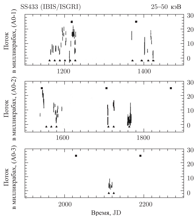
Рис. 134. Рентгеновские наблюдения SS 433 в 2003–2005 гг. По оси абсцисс — время, по оси ординат — рентгеновский поток в диапазоне 25–50 кэВ, выраженный в милликрабах. Темные квадраты вверх обозначают момент максимального раздвижения подвижных эмиссий ( T_3 ), темные треугольники вниз — момент середины рентгеновского затмения
