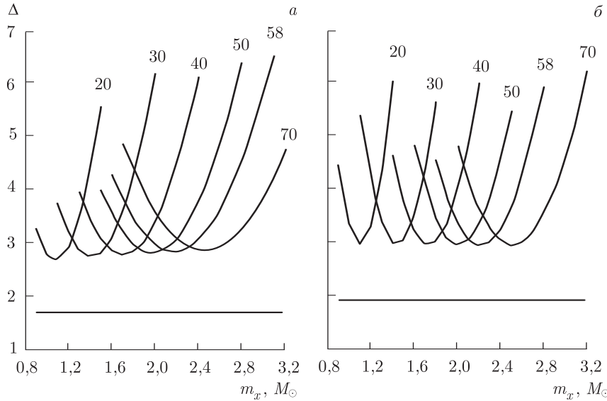
Рис. 183. Значения невязок, полученных методом 1, т. е. с использованием всех значений средней наблюдаемой лучевой скорости, между средней наблюдаемой кривой лучевых скоростей системы 4U 1700-37 и синтезированной кривой в модели Роша: a — по данным работы (Hammerschlag-Hensberger et al., 1978), горизонтальная линия соответствует критическому значению невязки в рамках статистики Фишера \Delta_{14,570} = 1,69 на уровне значимости \alpha = 5\% . Масса оптической компоненты, при которой получена невязка \Delta , указана около кривых в массах Солнца; b — то же, с использованием работы (Hammerschlag-Hensberger et al., 2003). Горизонтальная линия здесь соответствует критическому значению невязки в рамках статистики Фишера \Delta_{12,61} = 1,916 на уровне значимости \alpha = 5\%
