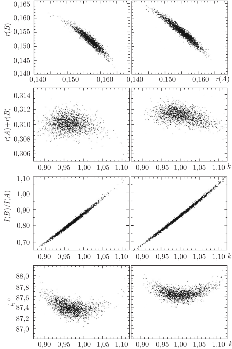
Рис. 84. Распределение наилучших оценок параметров системы WW Aug, полученное методом Монте-Карло (из работы Southworth et al., 2005a)
