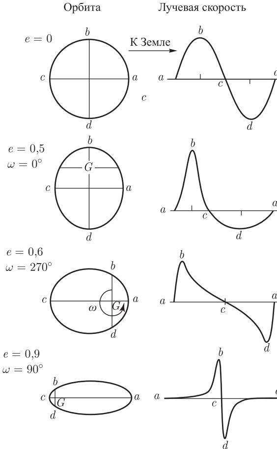
Рис. 2. Кривые лучевых скоростей при различных значениях элементов спектроскопической орбиты тесной двойной системы
