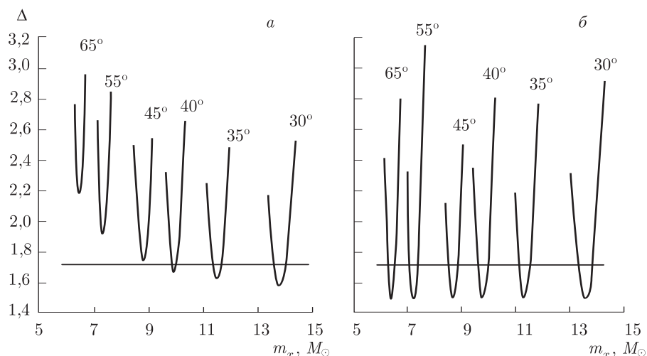
Рис. 162. a — невязки, полученные в процессе интерпретации средней наблюдаемой кривой лучевых скоростей системы Cyg X-1 в модели Роша методом 2 (без использования точек на кривой лучевых скоростей в фазах 0,4–0,6) при массе оптической звезды 22M_{\odot} для различных значений наклона орбиты i (приведены около кривых); б — то же для модели точечных масс
