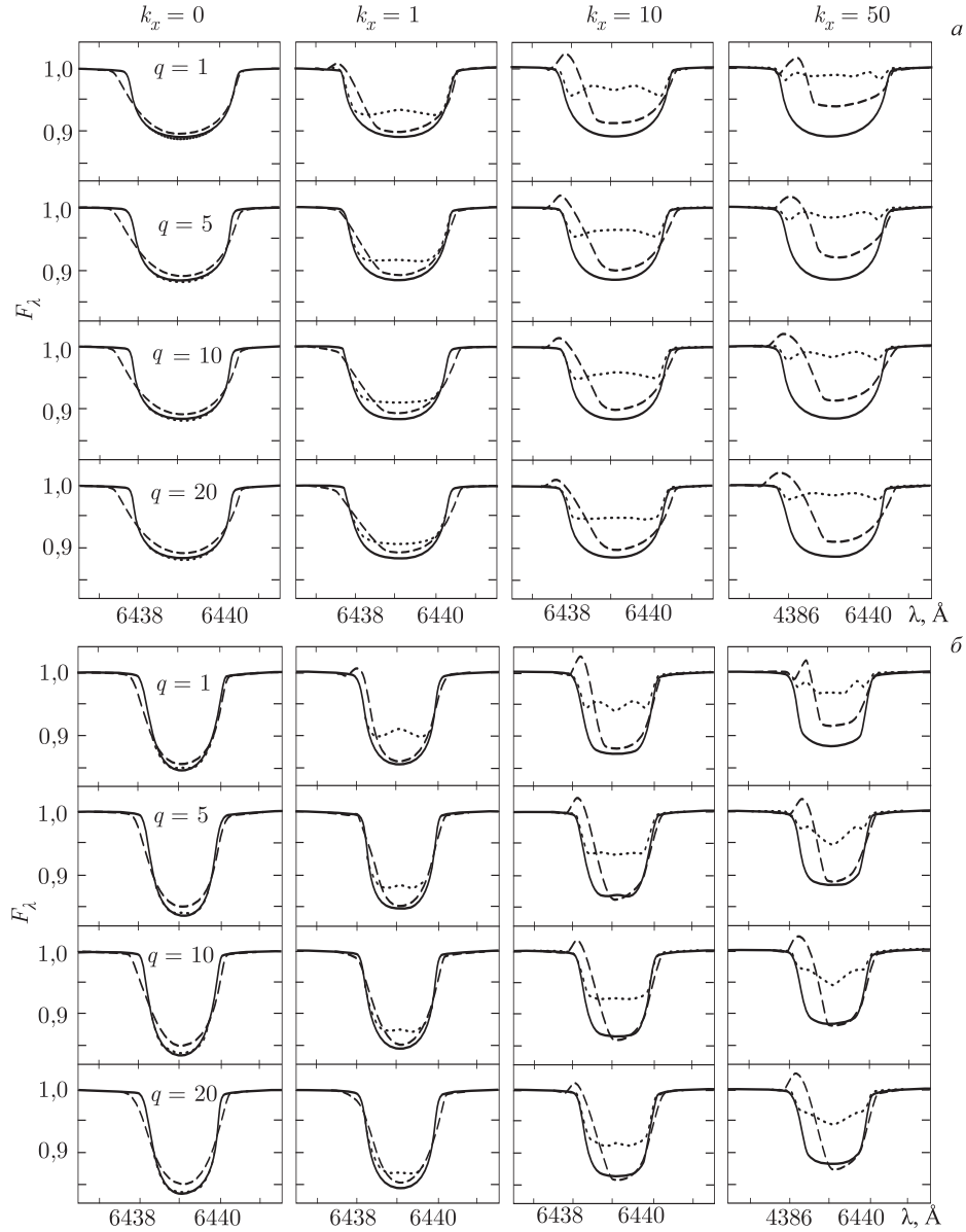
Рис. 61. Зависимость профилей линии Ca I 6439 Å от q и k_x для двух значений наклона орбиты i = 90^\circ (а) и i = 45^\circ (б). Параметры модели: q = 1-20 , k_x = 0-50 , \mu_v = 1 , T = 5000 К. Профили приведены для трех орбитальных фаз: сплошные линии — рентгеновский источник расположен сзади оптической звезды, штриховые — \varphi = 0,25 , звезда вида «сбоку», точечные линии — \varphi = 0,5 , рентгеновский источник впереди
