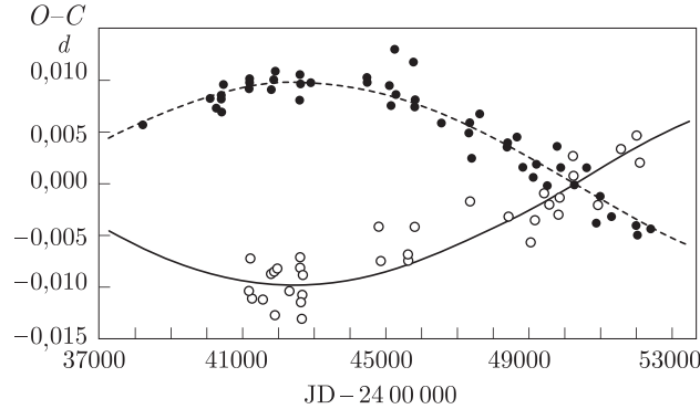
Рис. 19. Отклонения наблюдаемых ( O ) фотоэлектрических моментов минимумов системы HS Her от вычисленных ( C ) с линейными эфемеридами C(\text{MinI}) и C(\text{MinII}) соответственно для MinI (темные кружки) и MinII (светлые кружки) (из статьи Халиуллина и Халиуллиной, 2006)
