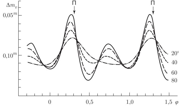
Рис. 50. Зависимость формы теоретической оптической кривой блеска рентгеновской двойной системы с эксцентрической орбитой при e = 0,12 и \omega_v = 31^\circ ( \psi_0 = 0,3 ) от значения наклона орбиты i , указанного цифрами на кривых. Стрелкой указан момент прохождения оптической звезды через периастр орбиты
