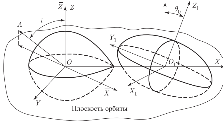
Рис. 48. Схематическая модель рентгеновской двойной системы с «прецессирующим» толстым аккреционным диском. Здесь OA — направление на наблюдателя (лежит в плоскости O\bar{X}Z ), OZ — нормаль к плоскости орбиты, O_1Z_1 — нормаль к экваториальной плоскости диска
