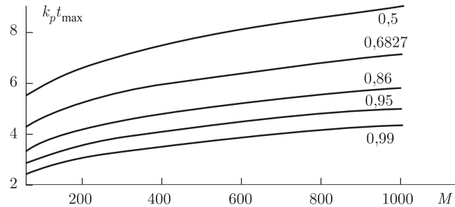
Рис. 39. Случай многопараметрической задачи. Параметр k_p t_{\max} для многопараметрической задачи в зависимости от числа наблюдаемых точек M и уровня доверия \gamma при P = 10 . Уровень доверия указан рядом с соответствующей кривой. Обращает на себя внимание то, что вероятность попадания истинного значения параметра в проекцию доверительной области, полученной в рамках статистики \chi^2_M , выше заданного уровня доверия \gamma = 0,6827 : она составляет \sim 0,80 . В то же время, вероятность попадания истинного решения в интервал ошибки, полученной в рамках метода дифференциальных поправок, равна заданному уровню доверия \gamma = 0,6827 . При этом вероятность одновременного попадания истинных значений параметров во все интервалы ошибок, полученных методом дифференциальных поправок, меньше заданного уровня доверия \gamma = 0,6827 (составляет \sim 0,5 )
