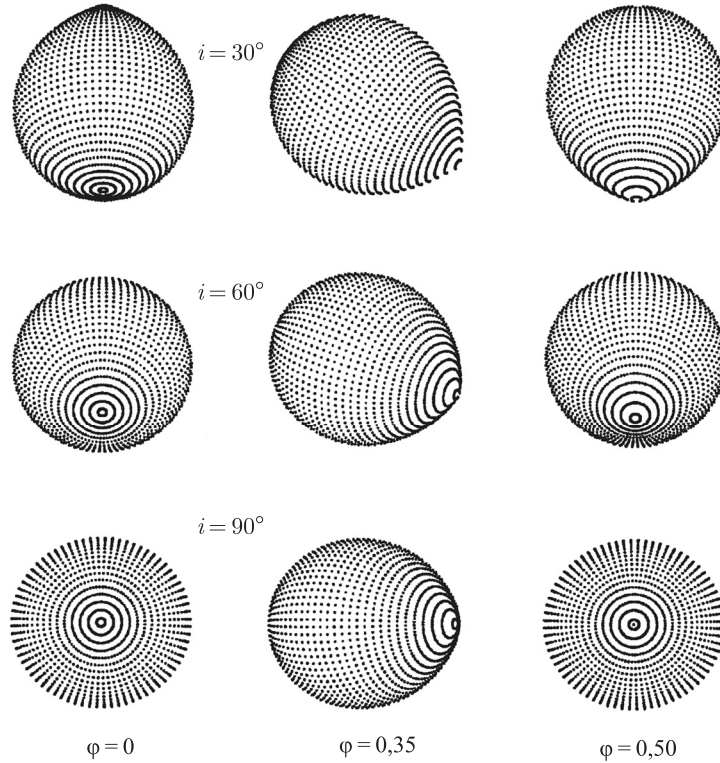
Рис. 156. Оптическая звезда рентгеновской двойной систем в модели Роша с q = 1 при степени заполнения полости Роша \mu=1 и наклоне орбиты i = 30^\circ, 60^\circ, 90^\circ в орбитальных фазах 0,0, 0,35, 0,5. При i = 90^\circ проекция звезды на картинную плоскость сильно меняется (от круговой формы, до грушевидной). «Носик» звезды, то затмевается, то нет, что приводит к заметному искажению профиля линии и кривой лучевых скоростей. При i = 30^\circ форма проекции звезды на картинную плоскость почти не меняется — меняется лишь позиционный угол фигуры, что не влияет на форму интегрального профиля линии и кривой лучевых скоростей
