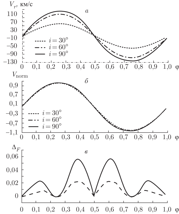
Рис. 152. а — теоретическая кривая лучевых скоростей оптической звезды с M_v = 20M_\odot , T_{\text{ef}} = 23000\text{ K} , вычисленная без учета влияния аппаратной функции на модельный интегральный профиль линии поглощения H_\gamma , при наклонении орбиты i = 30^\circ (пунктирная линия), 60^\circ (штрих-пунктирная линия) и 90^\circ (сплошная линия). Кривые лучевых скоростей рассчитаны с экспрессным алгоритмом (Антохина и Черепашук, 1994, Антохина, 1996), с использованием профилей линии H_\gamma в потоках из таблиц Куруца; б — те же кривые лучевых скоростей, нормированные на свое значение полуамплитуды лучевых скоростей для i = 30^\circ (пунктирная линия), 60^\circ (штрих-пунктирная линия) и 90^\circ (сплошная линия). в — разность модулей нормированных кривых лучевых скоростей \Delta_F = |V_{\text{norm}}(i = 90^\circ)| - |V_{\text{norm}}(i = 30^\circ)| (сплошная линия) и \Delta_F = |V_{\text{norm}}(i = 90^\circ)| - |V_{\text{norm}}(i = 60^\circ)| (штриховая линия). Величины \Delta_F указаны в единицах полуамплитуды кривой лучевых скоростей K_v
