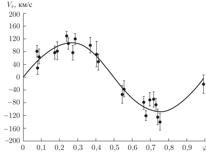
Рис. 195. Наблюдаемая и теоретическая кривые лучевых скоростей рентгеновской двойной системы M 33 X-7. Точки — значения лучевой скорости оптической звезды из работы (Orosz et al., 2007). Сплошная линия — теоретическая кривая лучевых скоростей в модели Роша, вычисленная при массе компактного объекта m_x = 15,55 M_\odot , массе оптической звезды m_v = 70 M_\odot и наклоне орбиты i = 74,6^\circ
