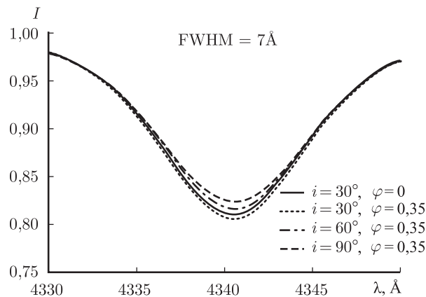
Рис. 155. То же, что на рис. 150, для случая учета влияния инструментального профиля с FWHM = 7 Å
