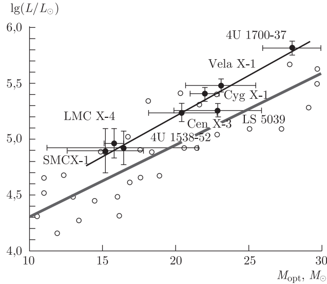
Рис. 161. Зависимость «масса–светимость» для ОБ-звезд в рентгеновских двойных системах (темные кружки) и ОБ-звезд, входящих в не взаимодействующие двойные системы, согласно работе (Неггеро, 1992) (светлые кружки). Серая линия — линейная аппроксимация методом наименьших квадратов зависимости для не взаимодействующих ОБ-звезд (Неггеро, 1992). Черной линией показана линейная аппроксимация для рентгеновских систем
