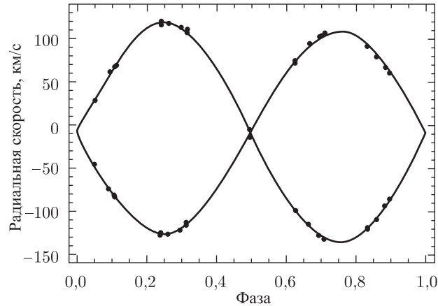
Рис. 82. Наблюдаемые и теоретические кривые лучевых скоростей затменной системы WW Aug (из работы Southworth et al., 2005a)
