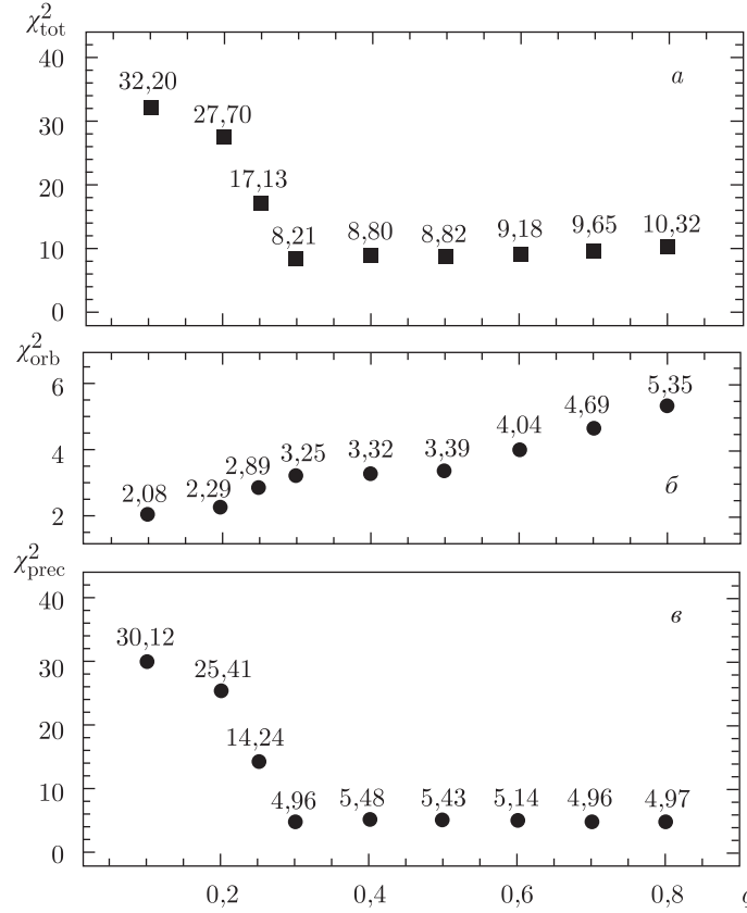
Рис. 145. a — суммарная невязка между наблюдаемой и теоретической кривой блеска, выраженная в виде приведенного хи-квадрат \chi^2_{\text{tot}} = \chi^2_{\text{orb}} + \chi^2_{\text{prec}} , где \chi^2_{\text{orb}} и \chi^2_{\text{prec}} — приведенные хи-квадрат для орбитальной (затменной) рентгеновской кривой блеска и прецессионной кривой блеска соответственно, как функция отношения масс компонент системы SS 433 q = m_x/m_v ; б — невязка \chi^2_{\text{orb}} — приведенное хи-квадрат для орбитальной кривой блеска как функция q ; в — невязка \chi^2_{\text{prec}} — приведенное хи-квадрат для прецессионной кривой блеска. Цифры около точек обозначают значения приведенного хи-квадрат
