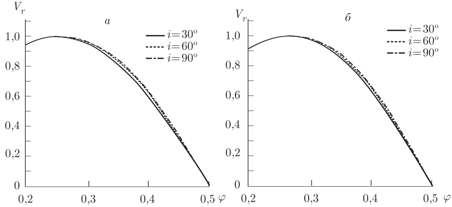
Рис. 165. Относительные теоретические кривые лучевых скоростей в модели Роша: a — при значениях m_v = 22M_\odot , m_x = 11,47M_\odot , e=0,0 для наклонений орбиты i = 30^\circ, 60^\circ, 90^\circ ; б — при значениях m_v=22M_\odot , m_x = 11,47M_\odot , e = 0,05 , \omega_v = 90^\circ для наклонений орбиты i = 30^\circ, 60^\circ, 90^\circ . Как и в случае круговой орбиты, видна зависимость формы кривой лучевых скоростей от наклона орбиты i при e \neq 0
