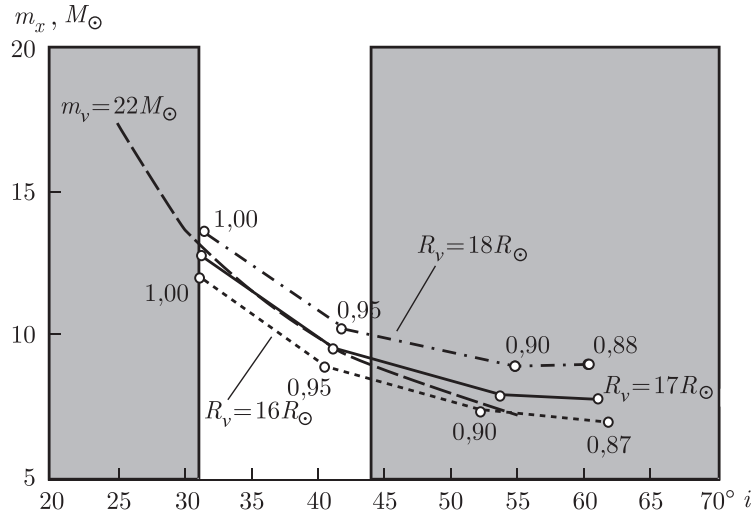
Рис. 160. Зависимость массы компактного объекта системы Cyg X-1 от наклона орбиты: сплошная линия получена из решения кривой блеска (Балог и др., 1981) при радиусе оптической звезды 17R_\odot (Herrero et al., 1995), штрих-пунктирная линия получена из решения кривой блеска (Балог и др., 1981) при радиусе оптической звезды 18R_\odot , пунктирная линия получена из решения кривой блеска (Балог и др., 1981), при радиусе оптической звезды 16R_\odot (Herrero et al., 1995), штриховая линия получена из наблюдаемой средней кривой лучевых скоростей при массе оптической звезды 22M_\odot . Цифры у светлых кружков показывают соответствующую величину степени заполнения полости Роша оптической звездой. Затемненные области соответствуют значениям i , неудовлетворяющим кривой блеска, приведенной в работе (Балог и др., 1981), и кривой лучевых скоростей
