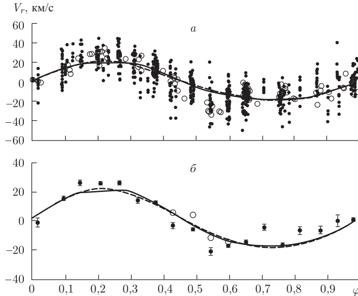
Рис. 171. а — сводная наблюдаемая кривая лучевых скоростей рентгеновской двойной системы Vela X-1. Здесь темными кружками представлены спектральные данные 1973 г. из работы (van Paradijs et al., 1977), светлыми кружками — спектральные данные 1995–1996 гг. из работы (Barziv et al., 2001). Для сравнения приведены теоретические кривые лучевых скоростей в модели Роша (сплошная линия) и модели точечных масс (штриховая линия) для массы m_x = 1,93M_\odot , соответствующей минимуму невязки в модели Роша. б — лучевые скорости, усредненные внутри фазовых интервалов (темными кружками представлена лучевая скорость, средняя в фазовом интервале, светлыми кружками — лучевые скорости, исправленные за нормированную функцию анизотропии звездного ветра оптической звезды). Для сравнения, приведена теоретическая кривая лучевых скоростей в модели Роша (сплошная линия) и модели точечных масс (штриховая линия) для m_x = 1,93M_\odot
