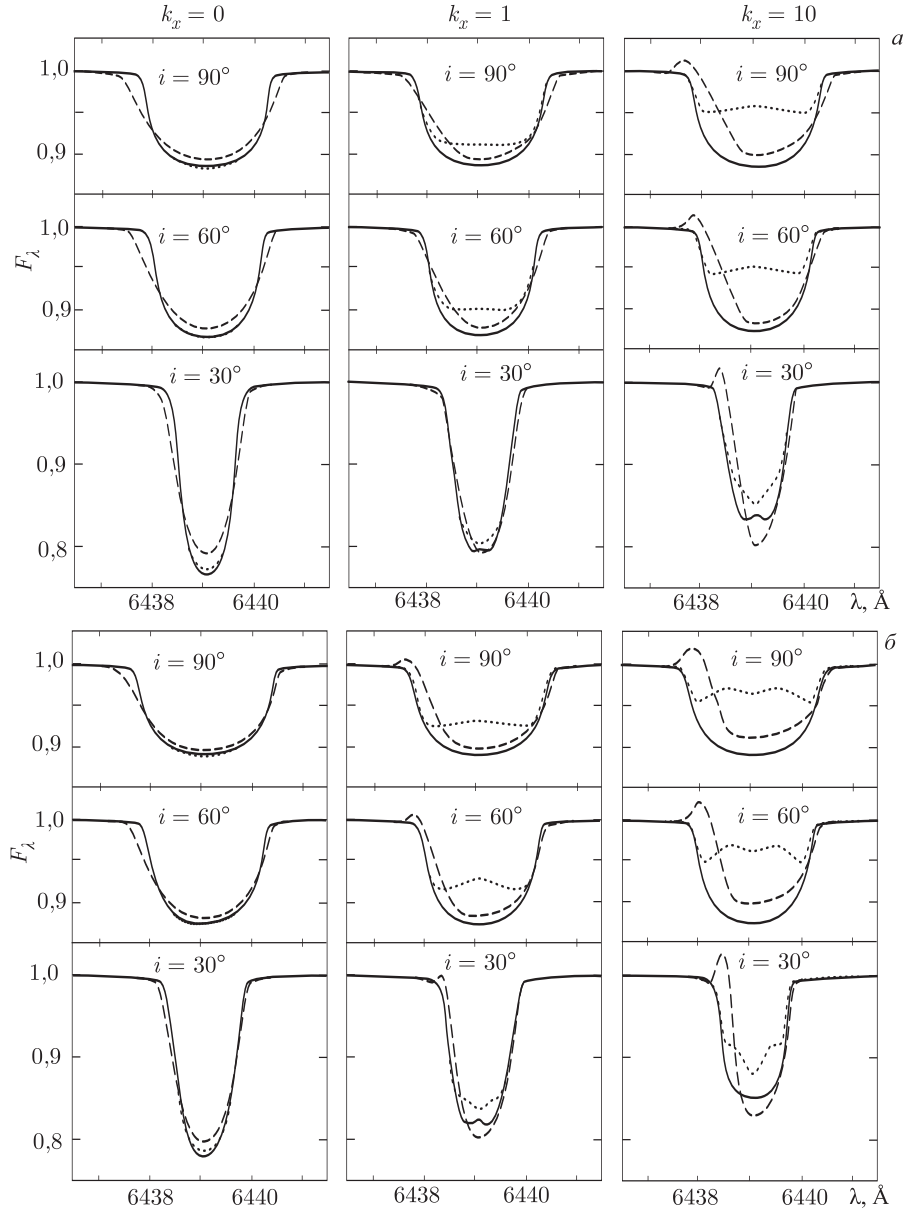
Рис. 62. Зависимость профилей линии Ca I 6439 Å от i и k_x для двух значений отношения масс q = 1 (а) и q = 10 (б). Параметры модели: i = 30-90 , k_x = 0-10 , \mu_v = 1 , T = 5000 K. Профили приведены для орбитальных фаз \varphi = 0 (сплошные линии), 0,25 (штриховые линии), 0,5 (точечные линии)
