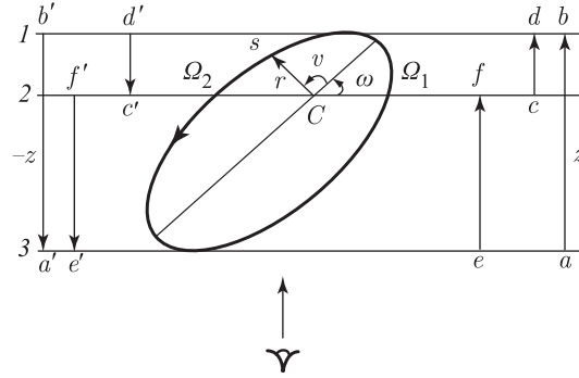
Рис. 4. Орбита одной из компонент спектрально-двойной системы, заключенная между двумя касательными плоскостями
