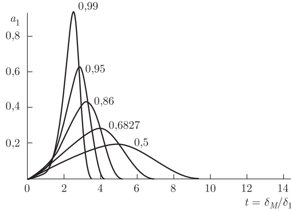
Рис. 36. Дифференциальная функция a_1(t) плотности распределения отношения величины доверительного интервала \Delta(\chi^2_M) , полученного на основе статистики \chi^2_M , при условии адекватности модели, к величине доверительного интервала, полученного методом дифференциальных поправок. Случай одномерной функции, M = 101 , \gamma = 0,5, 0,6827, 0,86, 0,95, 0,99
