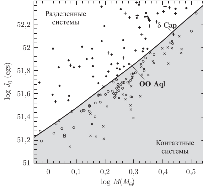
Рис. 88. Разделение контактных и разделенных систем на диаграмме «Суммарная масса–угловой орбитальный момент» (из работы Eker et al., 2006)
