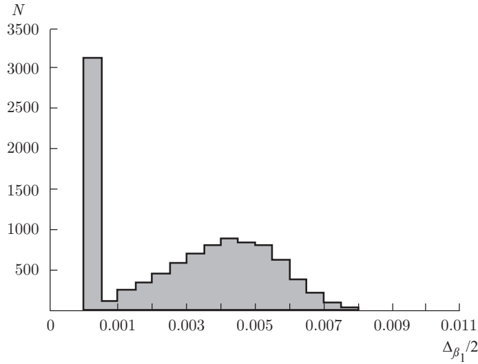
Рис. 26. Экспериментально полученная гистограмма плотности распределения полуширины доверительного интервала \Delta\beta_1/2 функции f(\theta, \beta_1) = \cos(\theta + \beta_1) + \sin \beta_1\theta . Интервалы получены в статистике \chi_M^2 в результате 10^4 испытаний. N — количество значений полуширины доверительного интервала \Delta\beta_1/2 , попадающих в соответствующий шаг гистограммы
