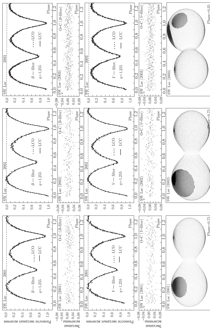
Рис. 86. Кривые блеска и соответствующие компьютерные модели системы типа W UMa SW Lac для разных эпох наблюдений: 2001 г. (слева), 2002 г. (в центре) и 2003 г. (справа) (из работы Albuja et al., 2004)
