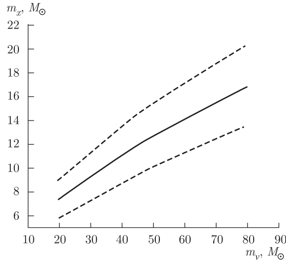
Рис. 201. Зависимость между массой компактного объекта m_x и массой оптической звезды m_v в системе М 33 Х-7, полученная в результате интерпретации наблюдаемой кривой лучевых скоростей из работы (Orosz et al., 2007) в модели Роша. Сплошная линия — центральные значения массы черной дыры, пунктирные линии соответствуют верхней и нижней границам ошибки центрального значения в рамках статистики \chi^2_M при уровне доверия \gamma = 95\% ( M — число наблюдаемых точек на кривой лучевых скоростей)
