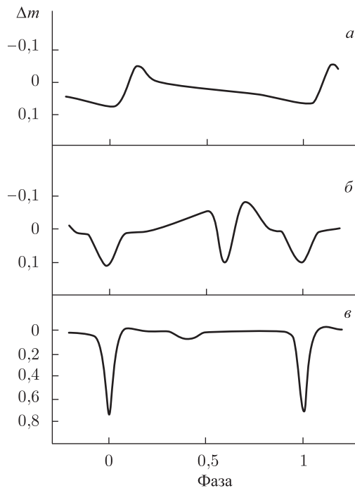
Рис. 57. Модельные теоретические кривые блеска для \lambda = 4400 \text{ \AA} . Соответствующие кривые лучевых скоростей приведены на рис. 56. В фазе 0,0 впереди находится первая звезда. Некоторые кривые имеют довольно необычную форму. Обратим внимание на различный масштаб по оси звездных величин первых двух графиков и третьего (сверху вниз)
