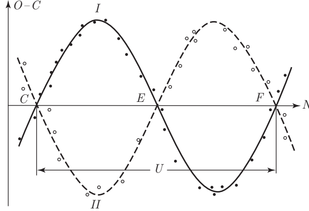
Рис. 16. Колебания остатков O - C , вызванные вращением линии апсид (Мартынов, 1971)
