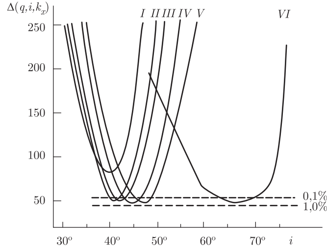
Рис. 126. Система XN Mus. Зависимость невязки \Delta от угла наклона орбиты i для различных значений q , \mu , k_x : I — q = 10 , эффект «отражения» не учитывается (в этом случае невязка больше, чем при учете эффекта отражения); II — q = 16 , \mu = 1 , k_x = 6 ; III — q = 10 , k_x = 5 ; IV — q = 5 , k_x = 3 ; V — q = 3 , k_x = 2 ; VI — q = 10 , \mu = 0,9 , k_x = 5 . Штриховыми линиями показаны критические значения невязки по уровню значимости 0,1% и 1% для статистики \chi^2
