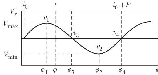
Рис. 6. Кривая лучевых скоростей с характерными точками
