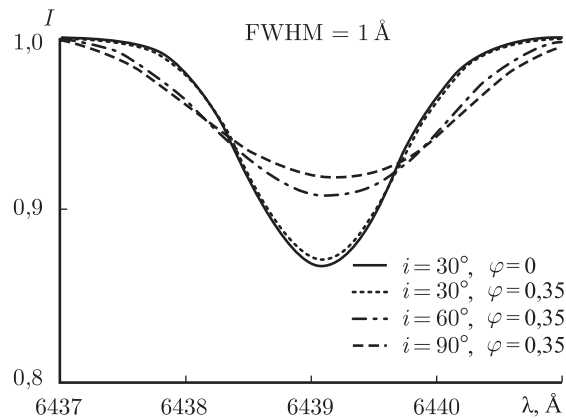
Рис. 154. То же, что на рис. 149, для случая учета влияния инструментального профиля спектрографа с FWHM = 1 Å
