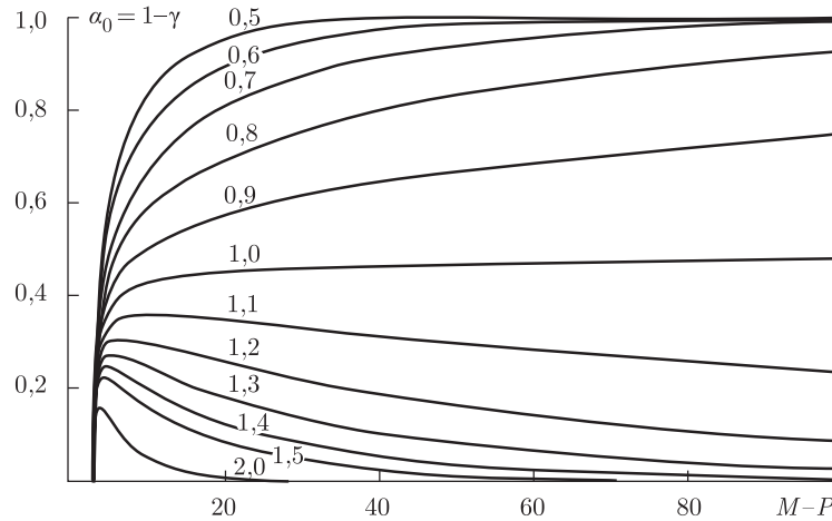
Рис. 40. Результаты решения уравнения \frac{\Delta_{M-P}(1-\alpha_o)}{M-P} = q относительно уровня значимости при P = 3 в зависимости от числа наблюдаемых точек M при заданном квантиле статистики приведенного \hat{\chi}_{M-P}^2 . Значение квантиля q указано рядом с соответствующей кривой. Видно, что когда минимальное значение приведенного хи-квадрат равно единице, соответствующий уровень значимости \alpha_o стремится к 0,5
