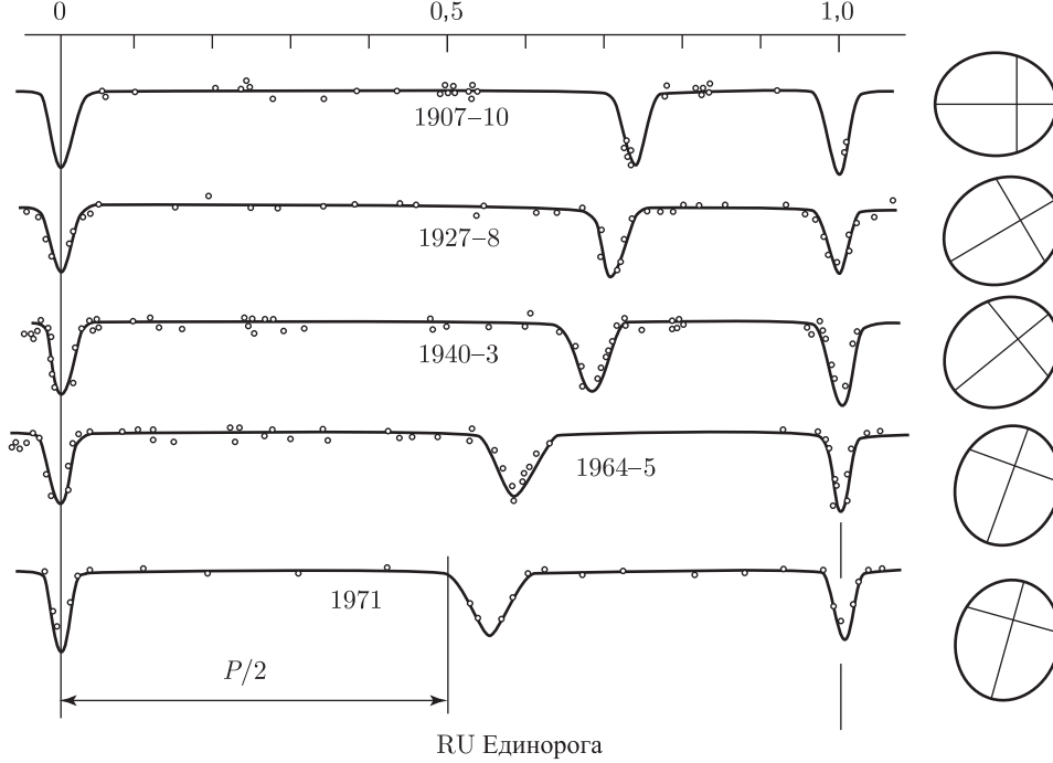
Рис. 15. Кривые блеска ТДС RU Моп за 1909–1971 гг., полученные Д. Я. Мартыновым, и соответствующий им поворот орбитального эллипса относительно наблюдателя
