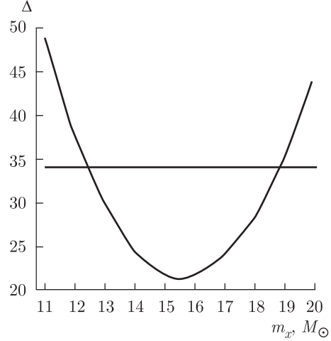
Рис. 200. Зависимость невязки \Delta в рамках статистики \chi^2_M между наблюдаемой и теоретической кривыми лучевых скоростей при m_v = 70 M_\odot . Горизонтальная линия соответствует критическому значению невязки на уровне значимости \alpha = 5\%
