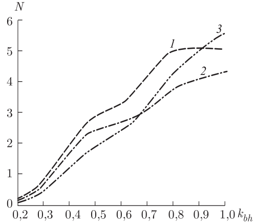
Рис. 204. То же, что на рис. 202 для системы типа IC 10 X-1
